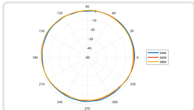
H-Plane: 3400 - 3800 MHz
