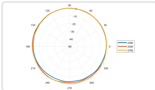
H-Plane: 2300 - 2700 MHz
